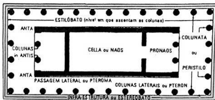
Planta (ao nível do pavimento) de um templo grego típico (segundo Grinnel)
